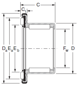
RAX 700
