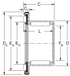
RAXF 700
